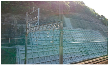
法面工事
